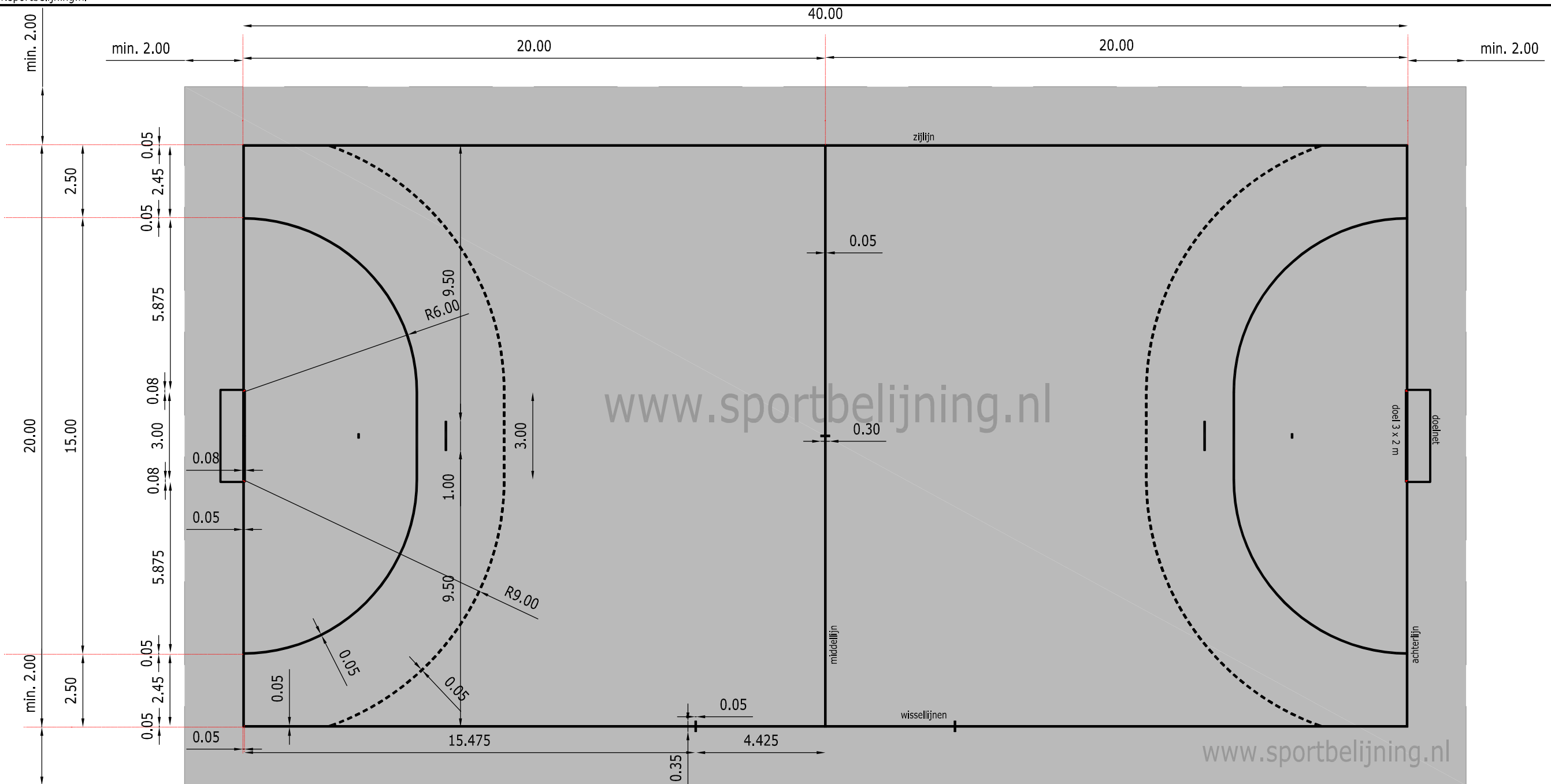
Schaal 1:150
