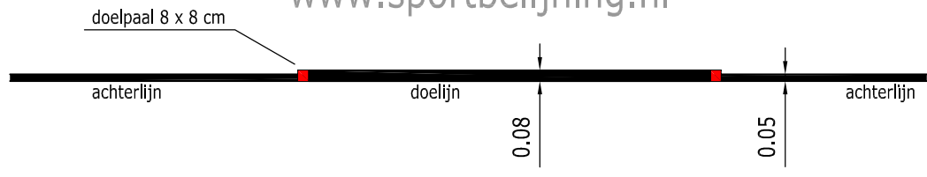
detail doellijn schaal 1:50
